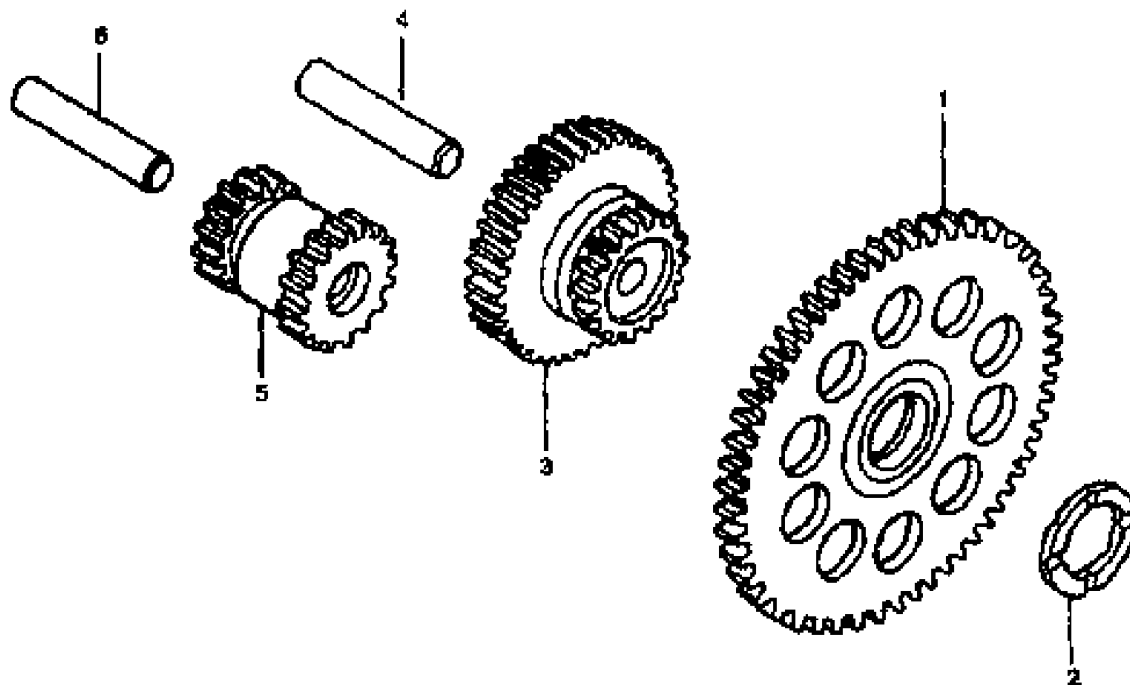
Рисунок 36 - Стартер
