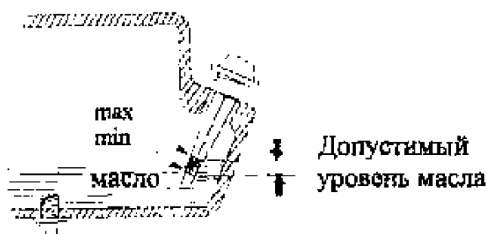
Рисунок 34 – Проверка уровня масла в картере
