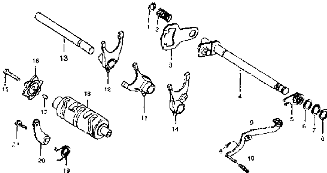
Рисунок 40 - Коробка передач
