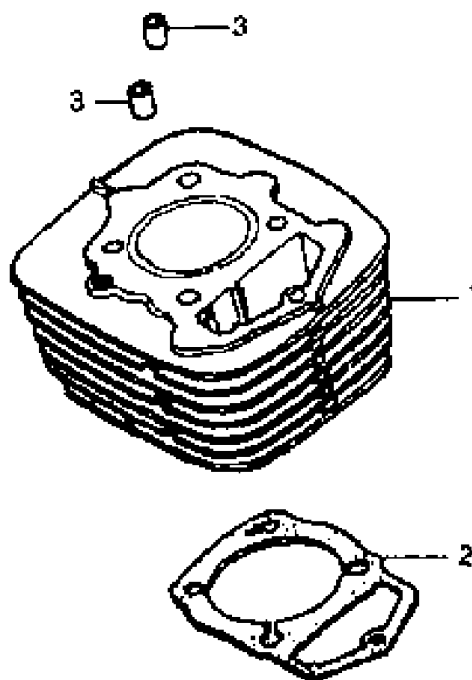
Рисунок 14 – Цилиндр
