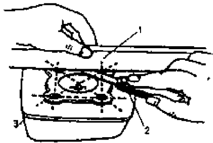
1-Линейка со шлифованными краями; 2-щуп; 3-головка цилиндра Рисунок 4 - Определение деформации поверхности
