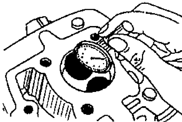
Рисунок 10 - Измерение внутреннего диаметра направляющей клапана
