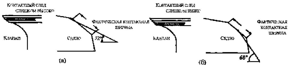
Рисунок 8 - Осмотр контактного следа на рабочей поверхности клапана после обработки шарошками
