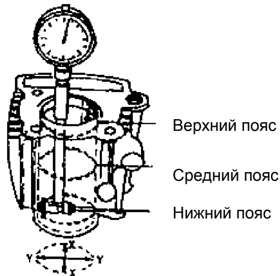
Рисунок 15- Измерение внутреннего диаметра цилиндра
