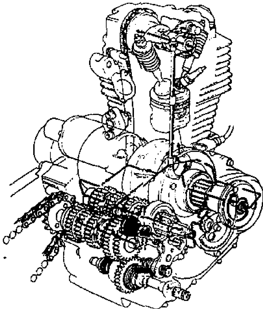
Рисунок 31 - Система смазки двигателя
